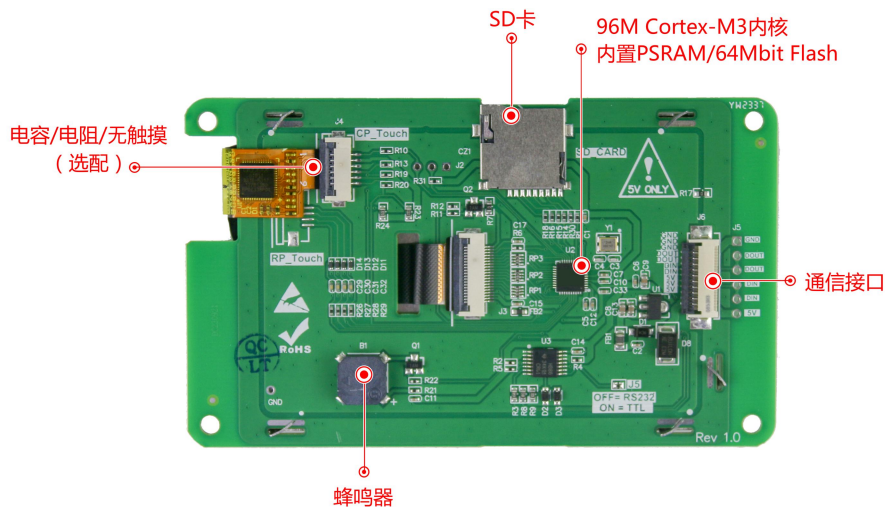
图 1-4 硬件配置图
