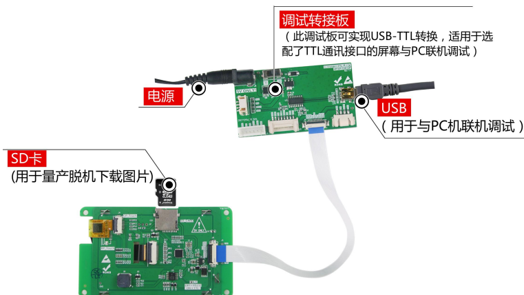
图 1-5 调试工具图
